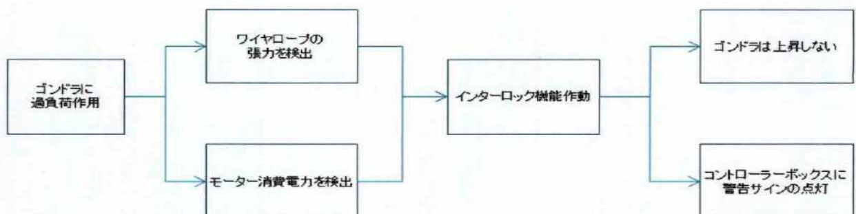
図4 過負荷制限装置フロー図
